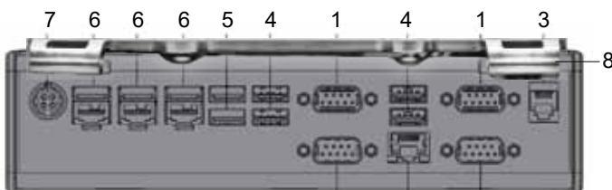
Module de ports externe
